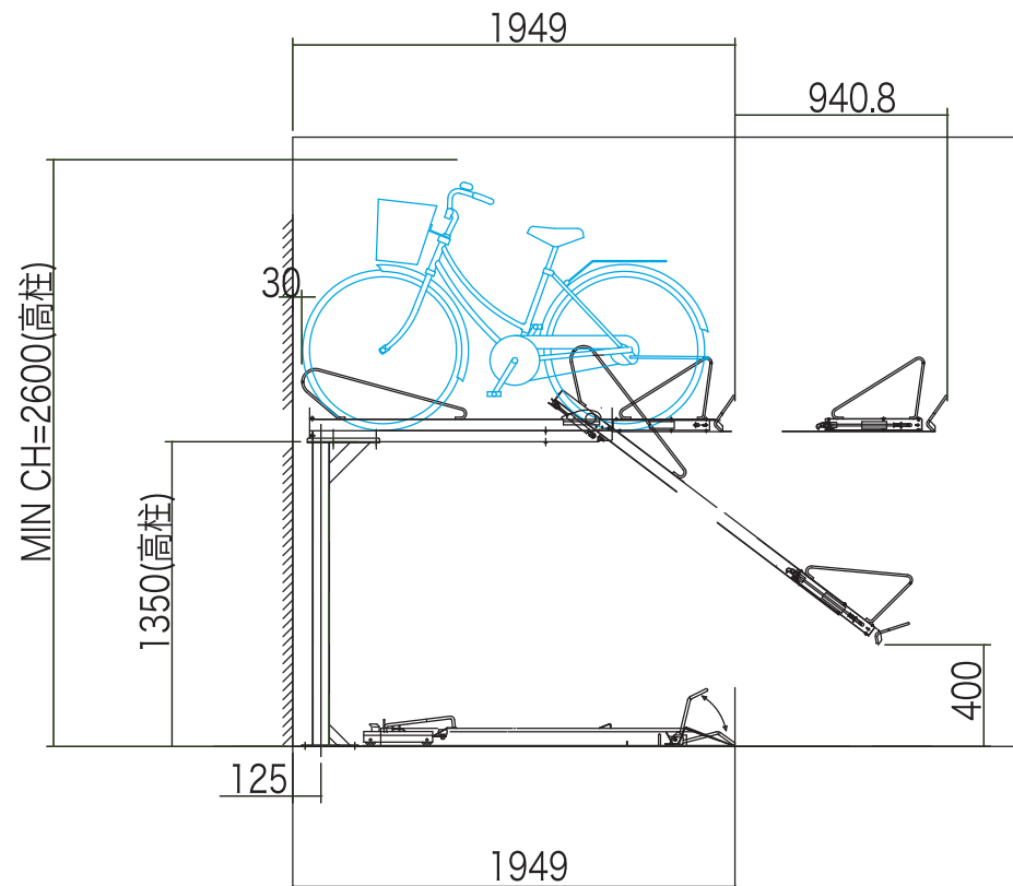
侧面图(高)
